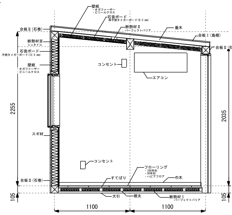
矩計図
